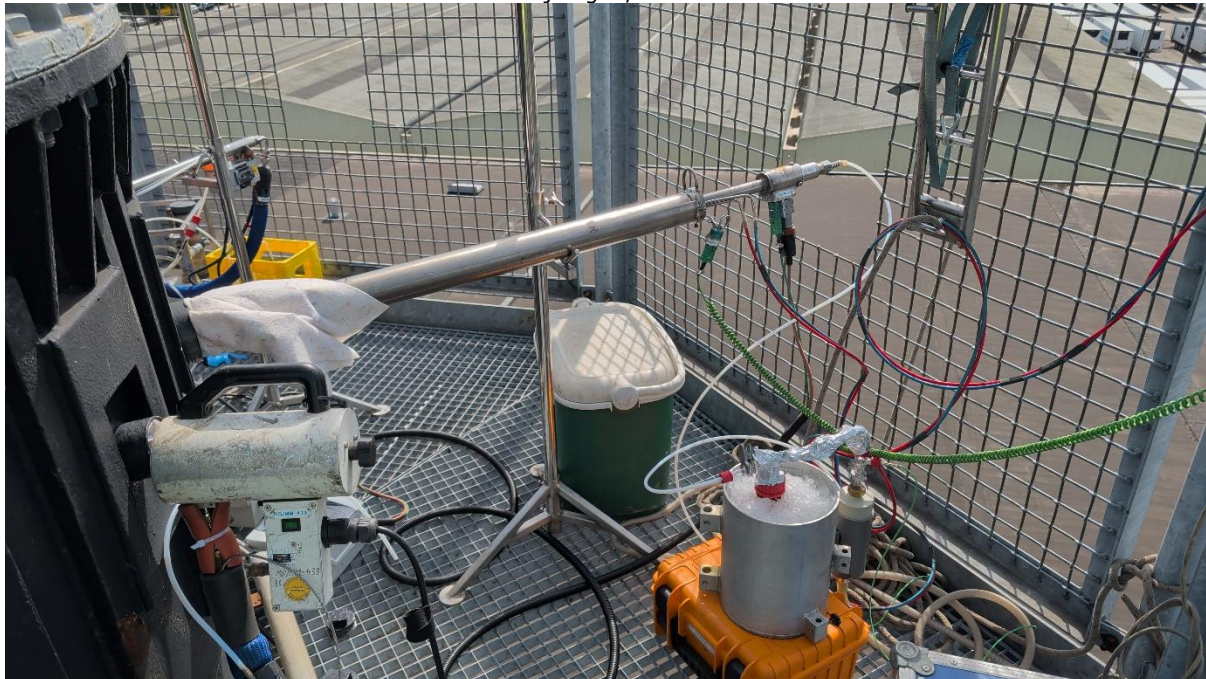
Foto 1c: Meetvlak centrale schoorsteen NIJG te Nijmegen, d.d. 7-7-2026.
