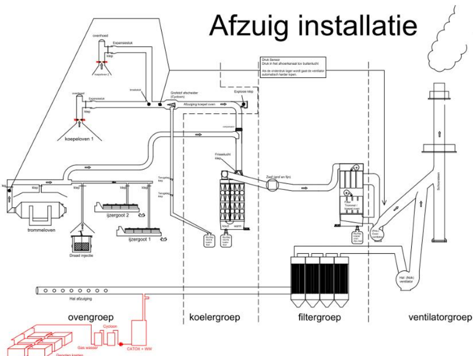
Figuur 3.1.1: Procesflowschema afzuigingen centrale schoorsteen de NIJG.
