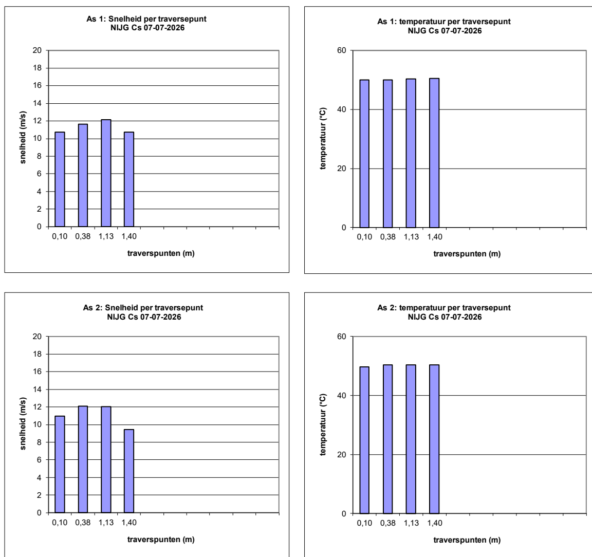
Figuur 1b: Resultaten beoordeling meetvlak centrale schoorsteen, d.d. 7-7-2026.
